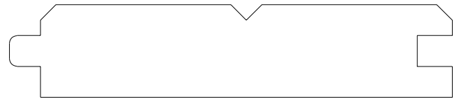
LM-X007 (3/4 X 3-9/16)
